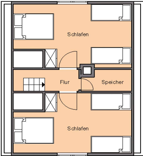
Obergeschoss
